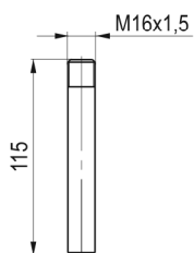
Удлинитель - Шток
